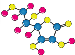
Ácido ascórbico o Vitamina C: C 6 H 8 O 6
